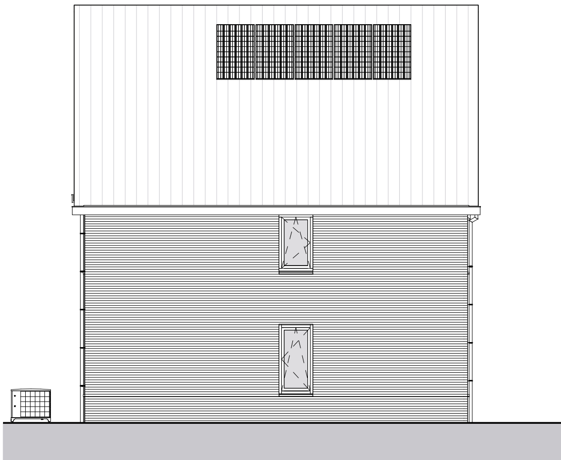
zijgevel
